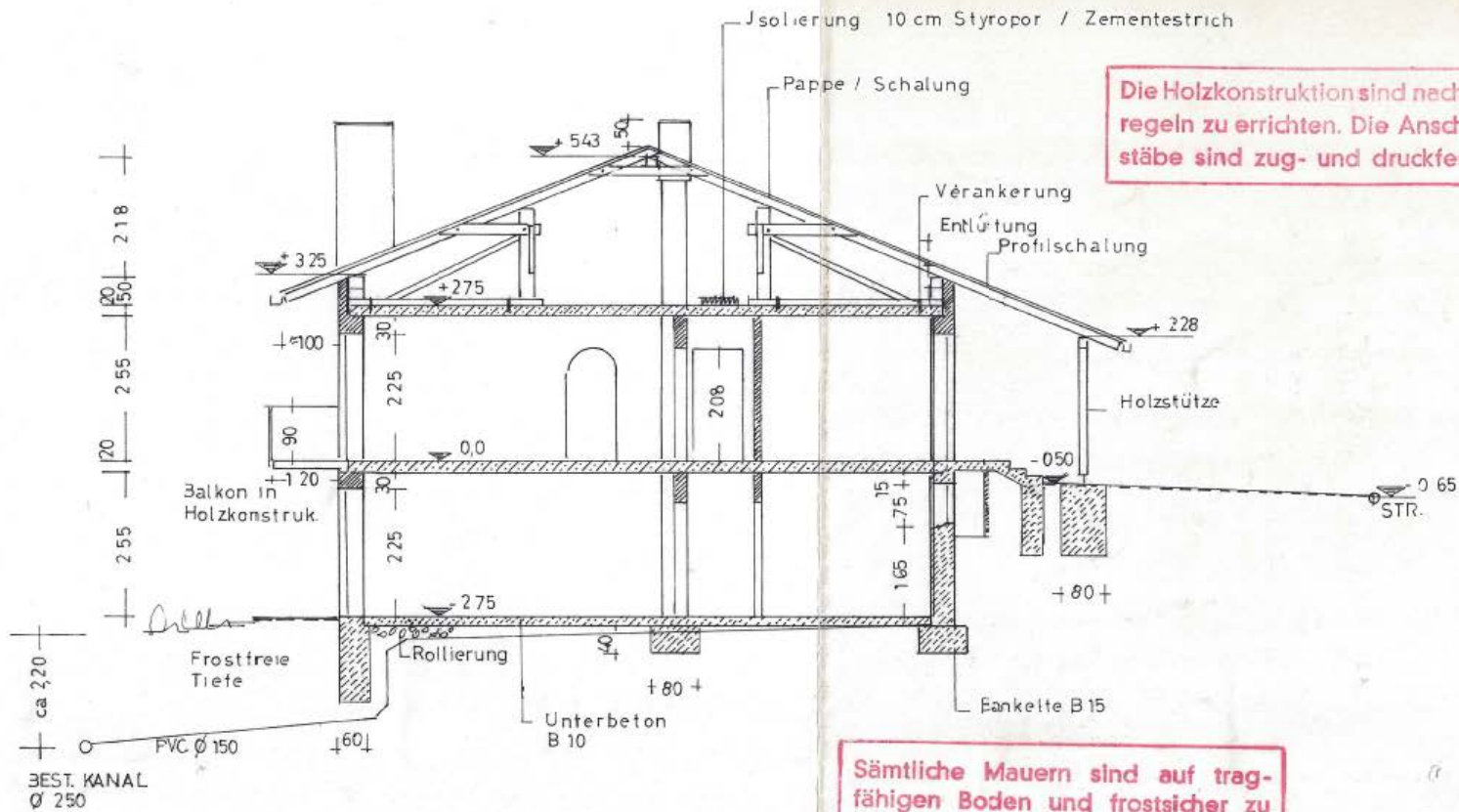
SCHNITT A - B
