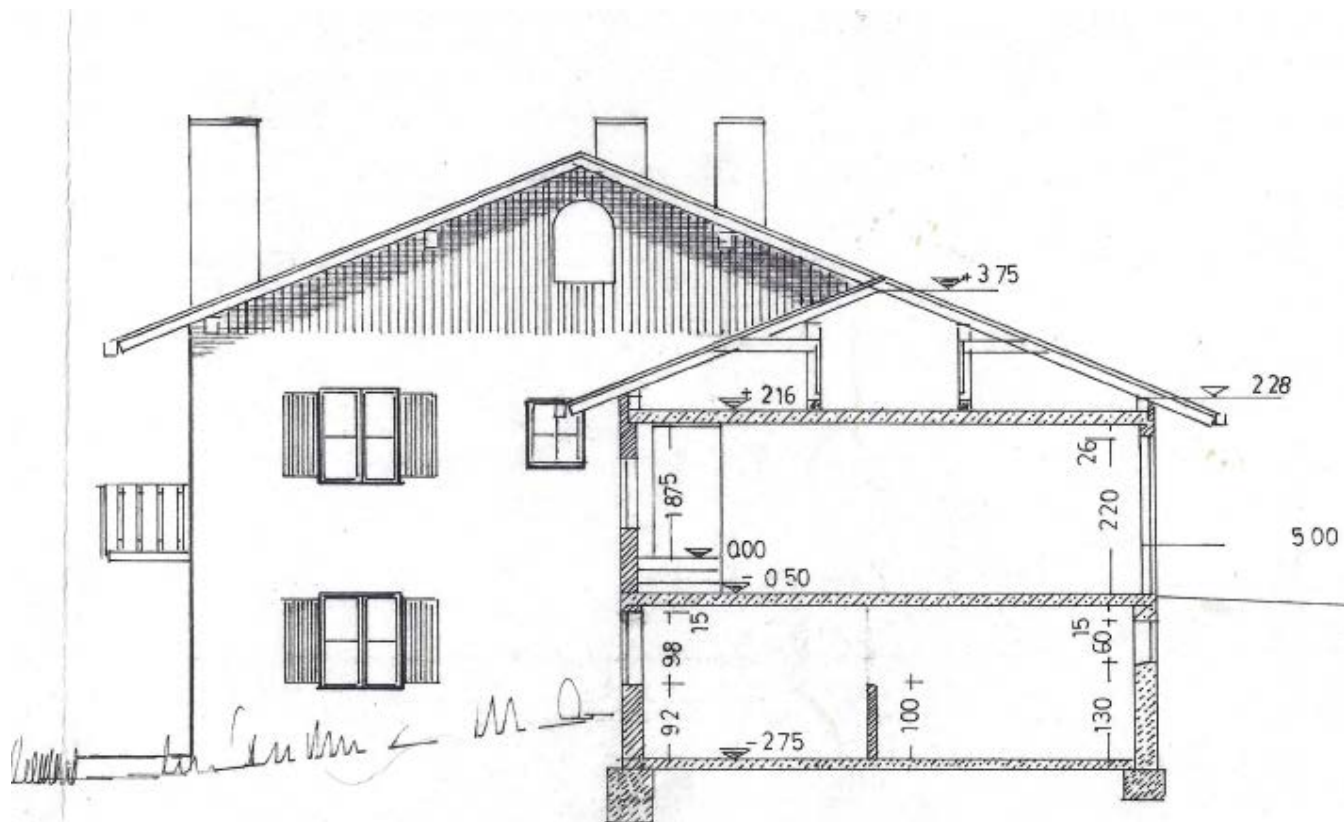
OSTANSICHT
