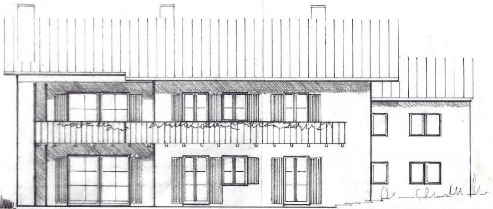
SÜDANSICHT
